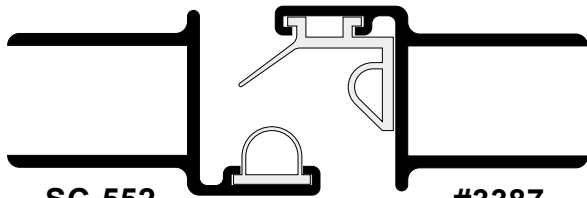
SC-552 64520 w/V-293 Pivot Jamb
