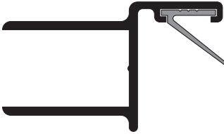
SC-552 64520 w/V-314 Strike Jamb
