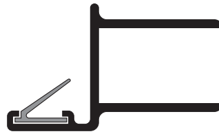
SC-552 64520 w/V-266 Hinge Jamb
