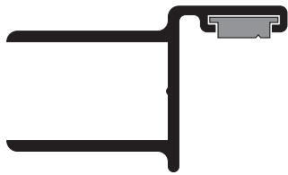
SC-552 64520 w/4033 Strike Jamb
